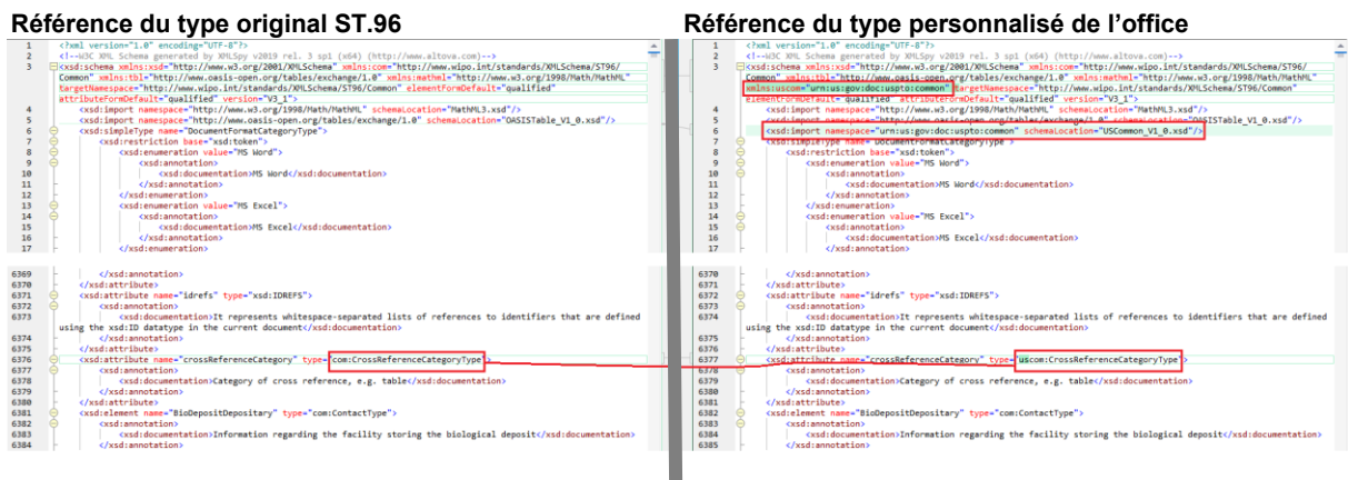
Figure 18 : Comparaison après application des règles de conception
