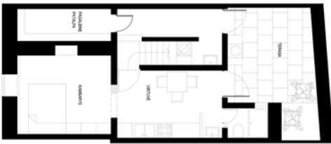
Buto architektūrinis projektas/brėžinys. Projekto autorė architektė Ugnė Purnaitė. Visos autoriaus teisės saugomos.
