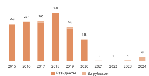
Патентные заявки *
